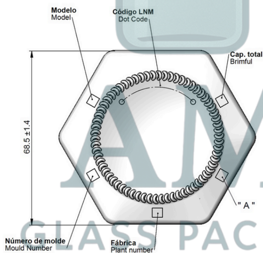
VISTA DO FUNDO BOTTOM VIEW
