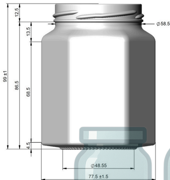
VISTA DE FRENTE FRONT VIEW
