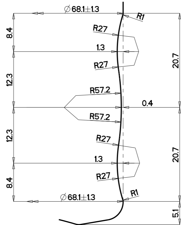
SECCIÓN / SECTION A-A ESCALA / SCALE 2/1
