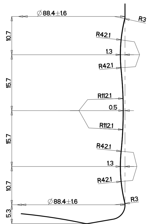
SECCIÓN / SECTION A-A ESCALA / SCALE 2/1
